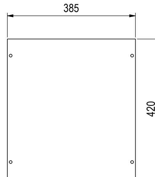
Montageplatte ( 1 : 7 )
