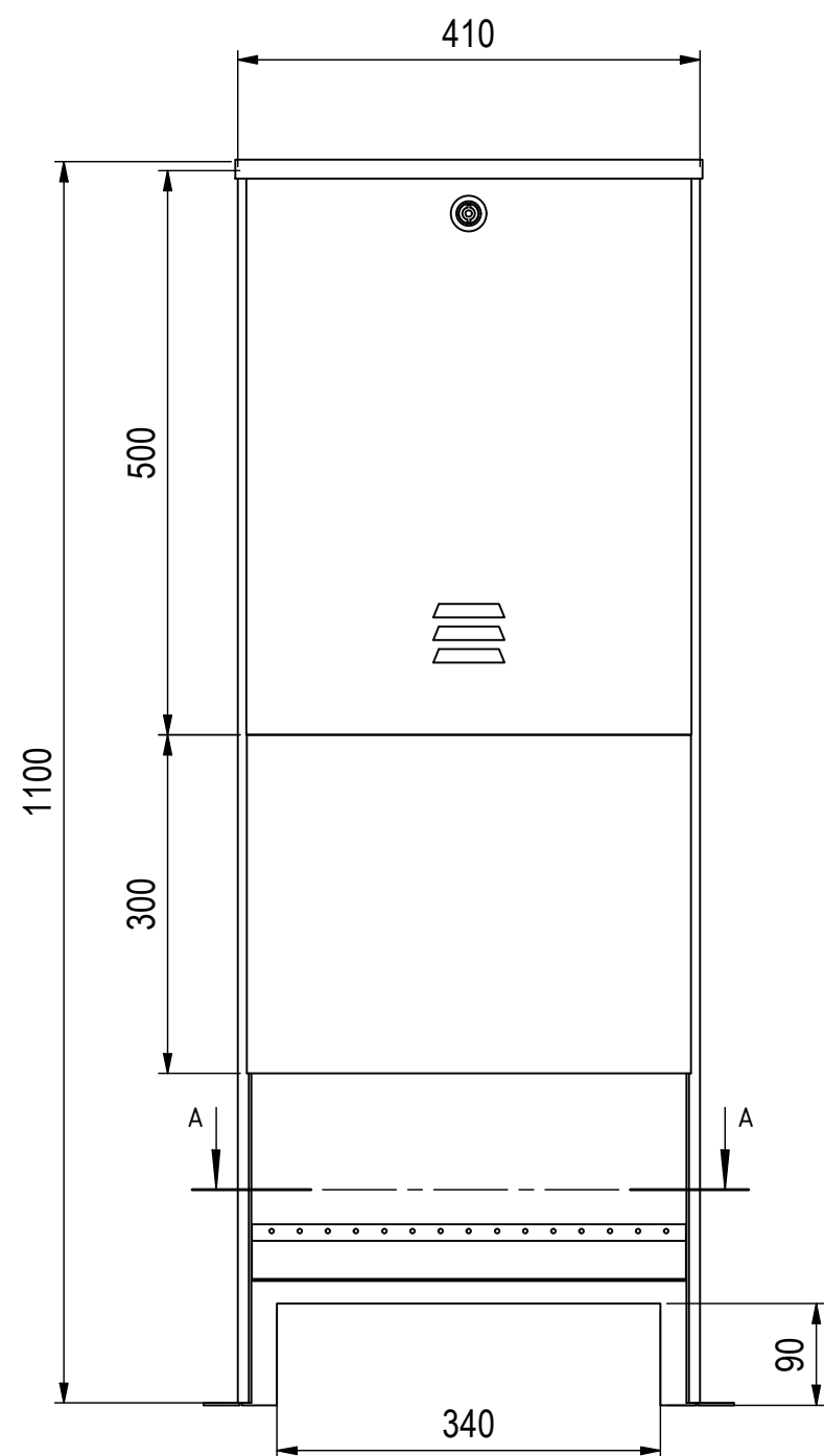
A-A ( 1 : 7 )
