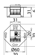
Maßbild DSA 230 LA
