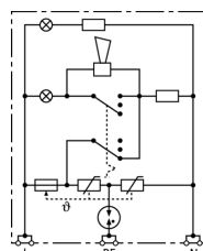
Prinzipschaltbild DSA 230 LA
