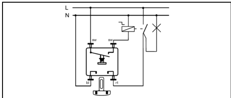
Anschlussbeispiel 534 U
