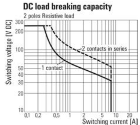
Ohmsche Last
