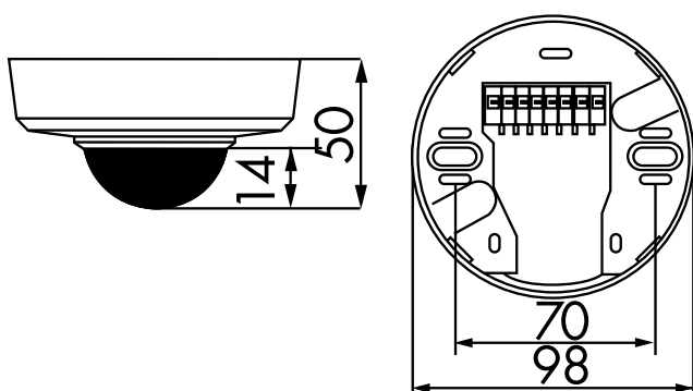
Bemaßung AP
