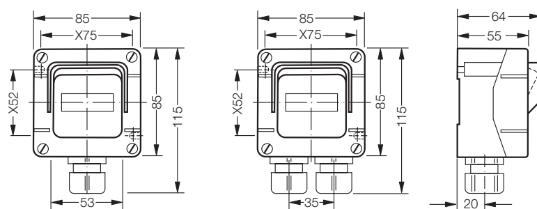
Schalter/Drucktaster
