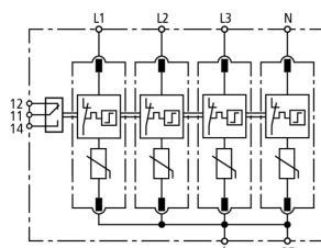
Prinzipschaltbild DG M TNS 275 FM
