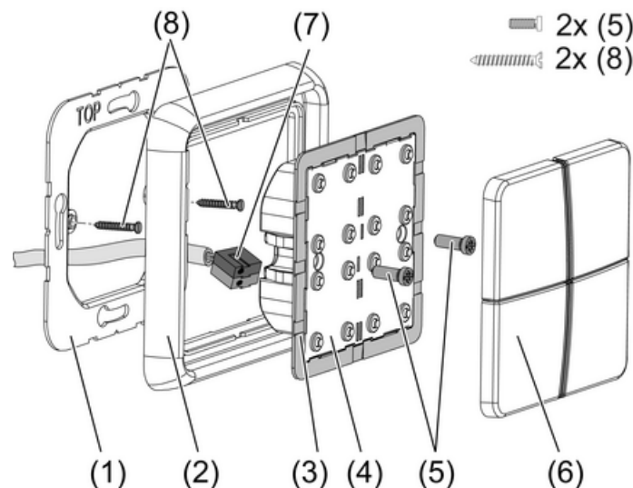
Bild 1: Montage Tastsensor-Modul
