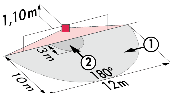
Reichweitendiagramm
