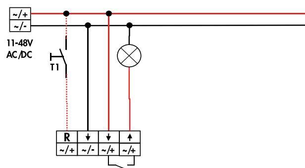
Schaltbild
