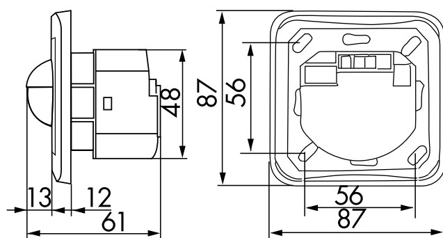
Bemaßung
