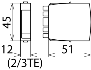
Maßbild BXT ML2 BD S 24
