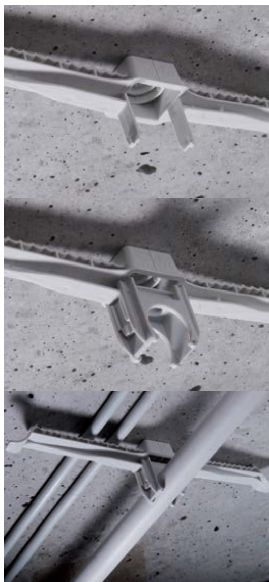
Mit Hilfe eines EC Euro-Clips lässt sich auch ein Rohr am KBS mittig befestigen.
