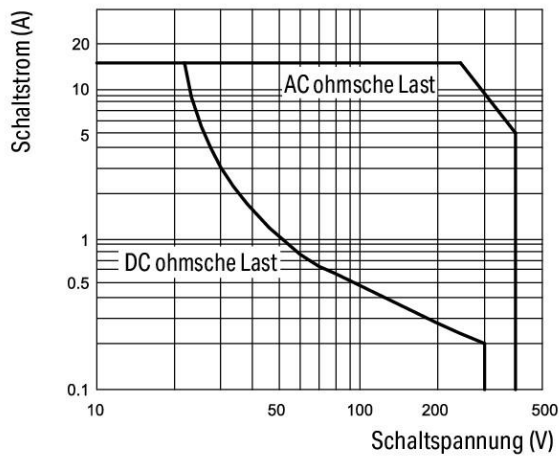
Lastgrenzkurve
