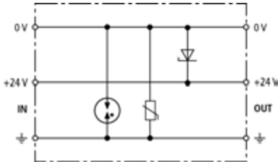
Prinzipschaltbild BVT AVD
