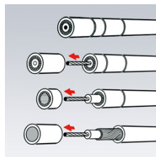
Dreistufige Abisolierung eines Koax-Kabels
