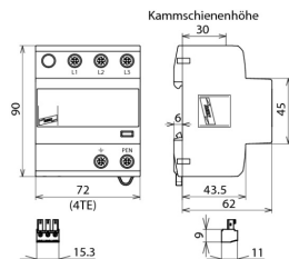
Maßbild DSH TNC 255 FM
