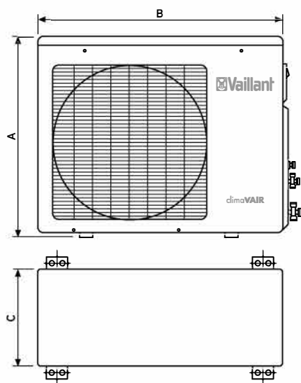
Außeneinheit
