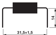
Maßzeichnung
