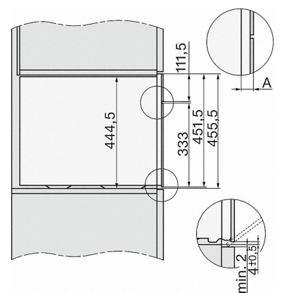
DG7x4x, DGM7x4x, DG7x4x-55, DGM7x4x-55, Skizze
