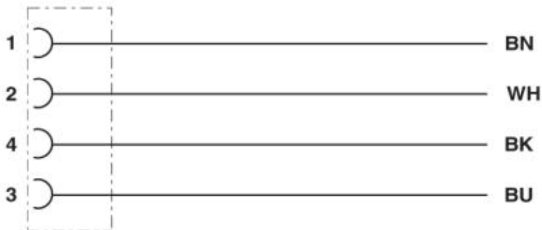
Schaltplan
