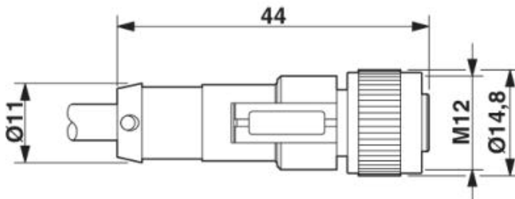
Maßzeichnung
