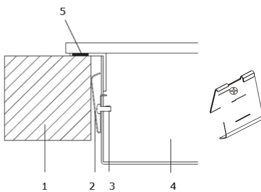
Abbildung 6 Glaskeramikkochfeld
