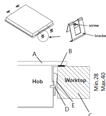
Abbildung 7 Querschnitt eingebautes Glaskeramikkochfeld
