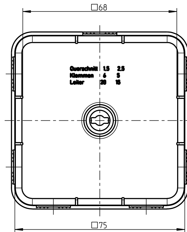
Innenansicht Deckel
