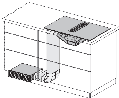
KMDA 7774, Einbauvariante 1 (Skizze)
