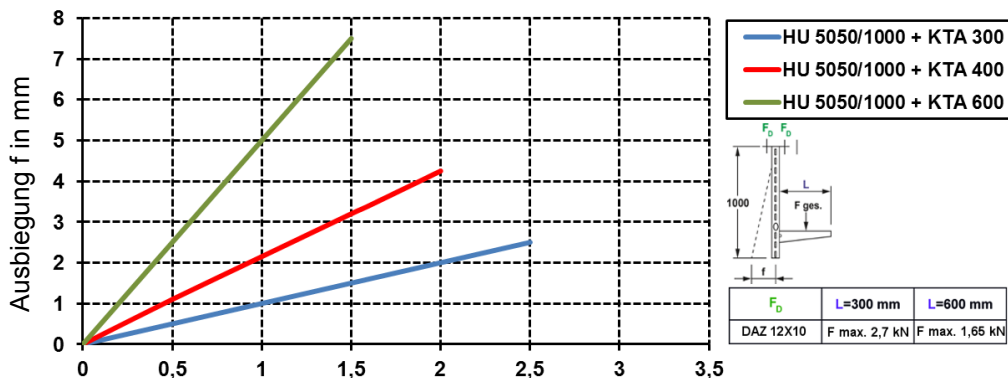
Belastungsdiagramm: Hängestielausbiegung bei einseitiger Lasteinleitung
