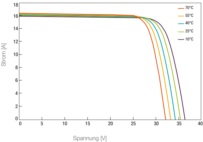
Strom-Spannungskurve des PV-Moduls in Abhängigkeit der Temperatur
