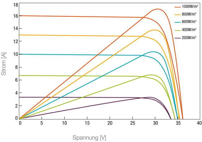
Strom-Spannungskurve des PV-Moduls in Abhängigkeit der Sonneneinstrahlung
