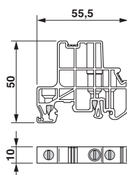
Maßzeichnung
