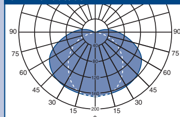
Lichtstärkeverteilungskurve eLLK 92058/58
