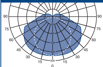
Lichtstärkeverteilungskurve eLLK 92018/18 / eLLK 92036/36
