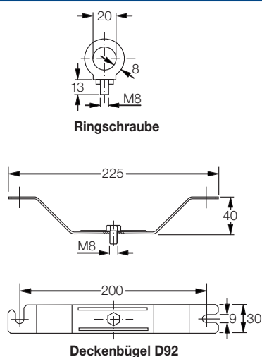
Deckenbügel D92
