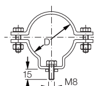
Rohrschelle
