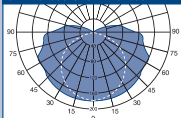
Lichtstärkeverteilungskurve eLLK 92036 / eLLK 92058
