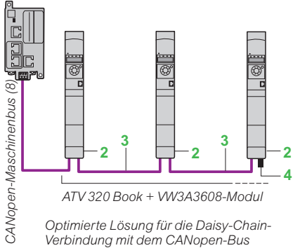
Modicon M251 (7)
