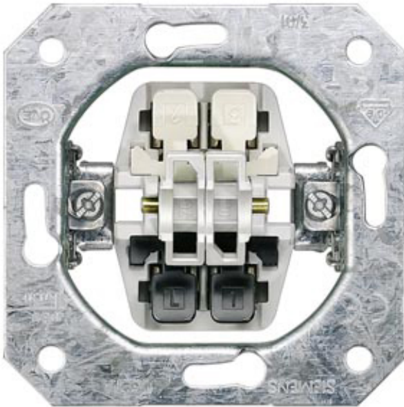
DELTA TASTER-GERAETEEINSATZ UP, JALOUSIETASTER 10A 250V ELEKTRISCH VERRIEGELT
