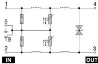
Prinzipschaltbild
