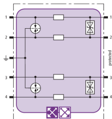
Principalschaltbild BXT ML4 BD HF 24
