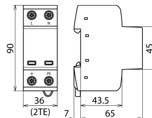
Maßbild DSH TN 255
