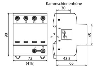
Maßbild DSH TT 255
