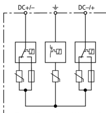
Prinzipialschaltbild DG YPV SCI 1000
