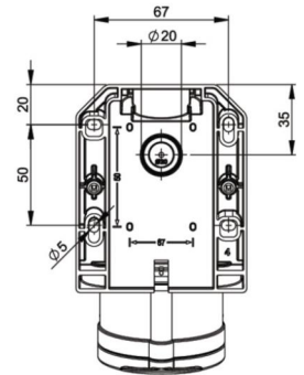
b=Höhe/height Neigung/angle=15°
