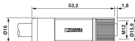
Maßzeichnung
