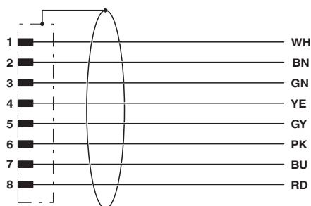
Kontaktbelegung des M12-Steckers
