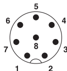
Polbild M12-Stecker, 8-polig, Ansicht Stiftseite
