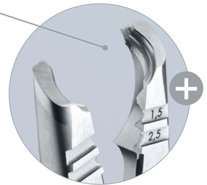
Rundschneide mit Tiefenbegrenzung: zum leichten und beschädigungsfreien Abmanteln
