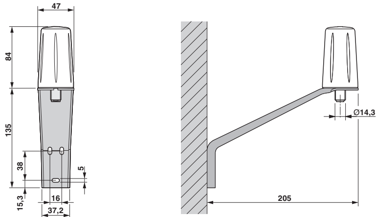
Maßzeichnung
